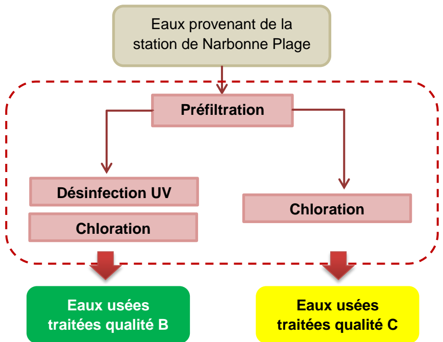
Prototype initial de Traitement tertiaire (1,5 m3/h)
